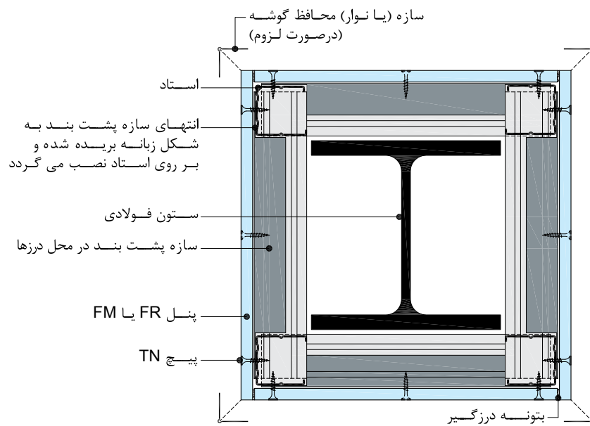
پوشش محافظ ستون - تک لایه (مقطع سازه‌های پشتیبان)
