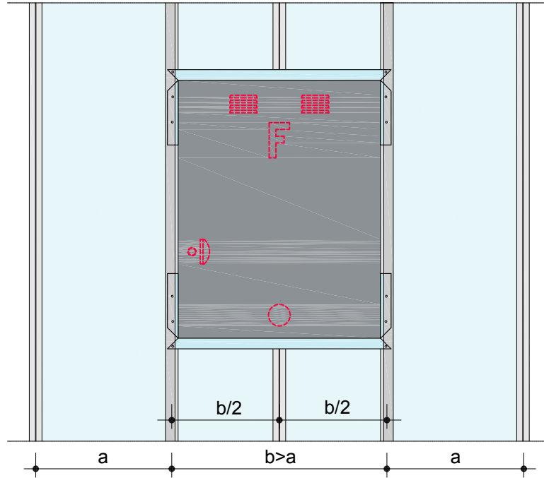
W-MI-A10 جزئیات قاب بندی در محل نصب جعبه آتش نشانی
